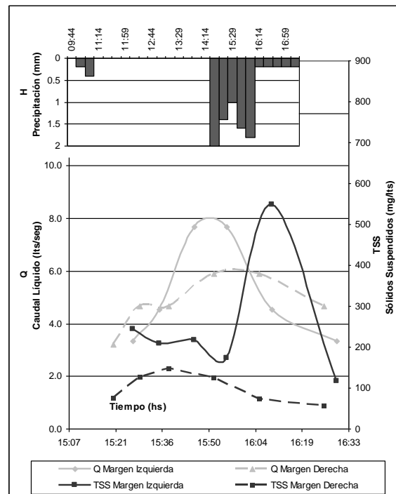
Figura 6. Hietograma, Hidrogramas y Polutogramas del Evento 5 (08/02/2010)
