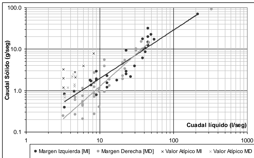
Figura 10. Curva Clave de Sedimentos de los afluentes a los sumideros de margen izquierda y derecha
