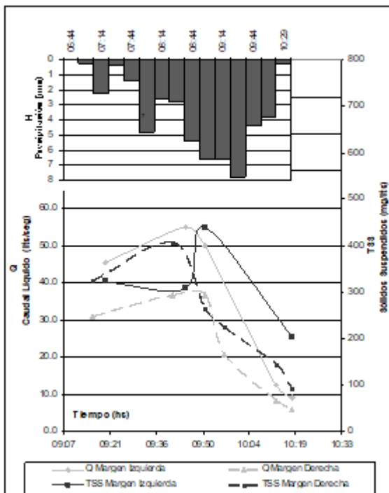
Figura 5. Hietograma, Hidrogramas y Polutogramas del Evento 3 (06/11/2009)
